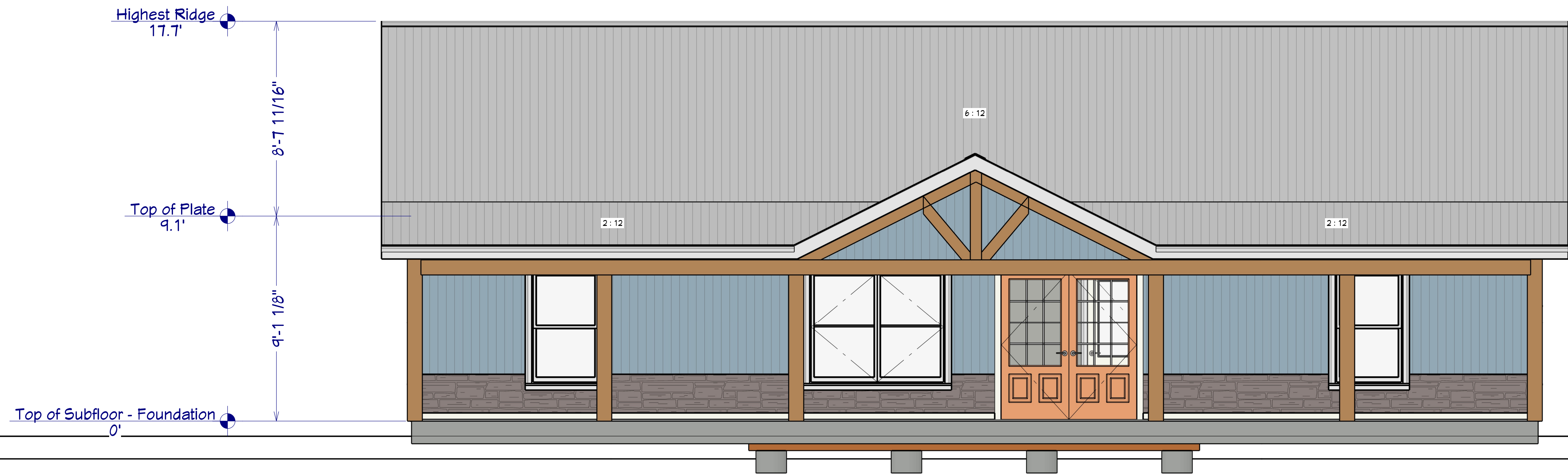
Elevation 5
